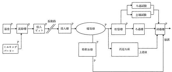
図-1 尿処理施設フロー図
